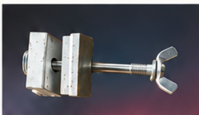
PIEZA DE UNIÓN ENTRE MARCOS (REFERENCIA PU-01)
